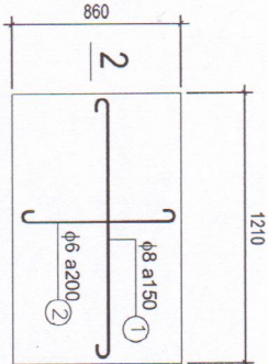
TẦM ĐÀN D2 (SL = 01C.K) TỈ LỆ : 1/25
