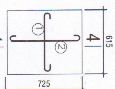
TẦM ĐÀN D4 (SL = 01C.K) TỈ LỆ : 1/25
