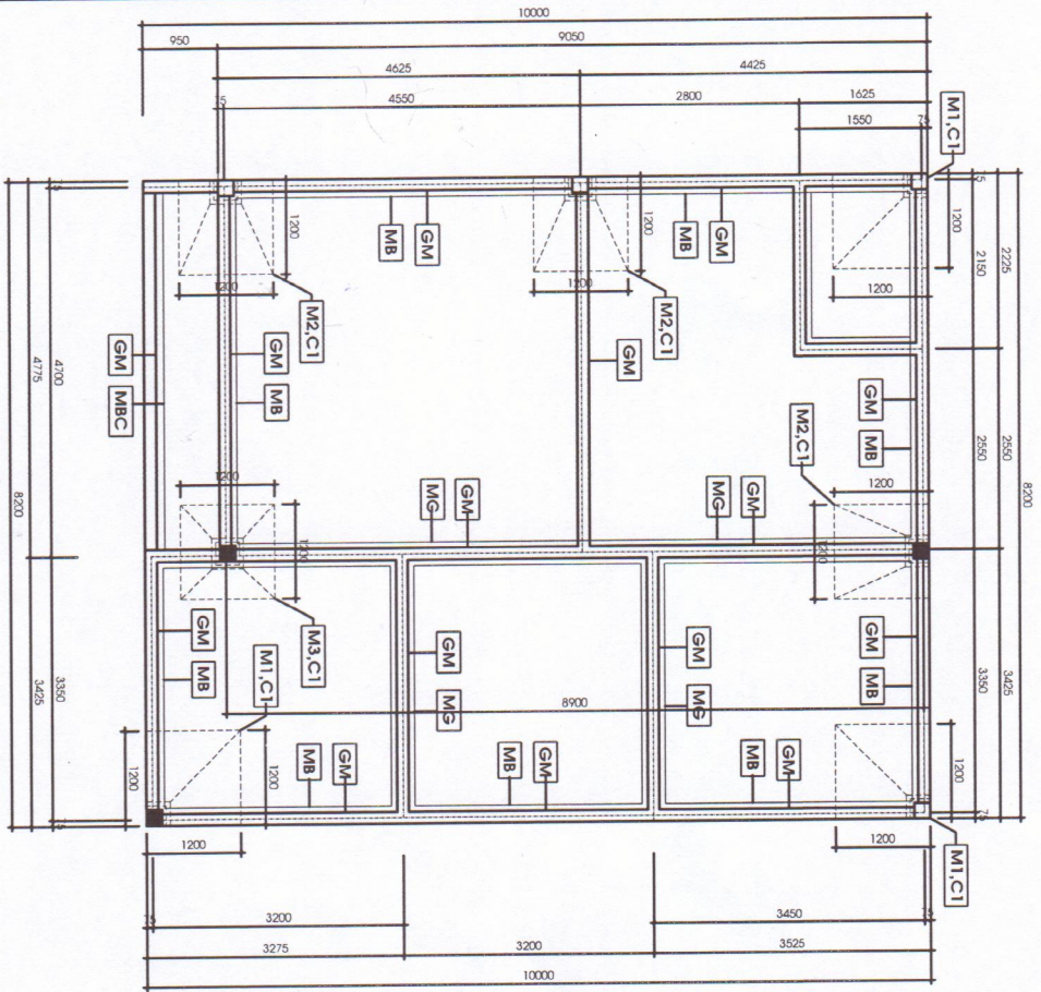
MẶT BẰNG MÓNG TỈ LỆ: 1/50
