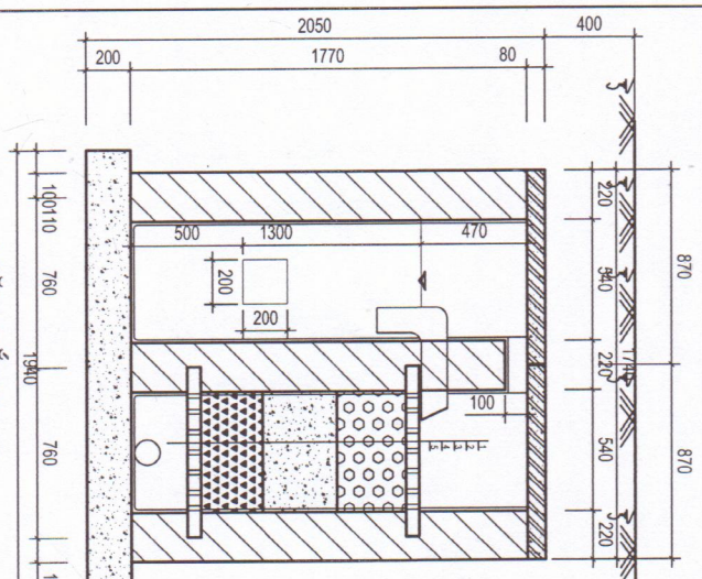
MẶT CẮT B - B TỈ LỆ : 1/25
