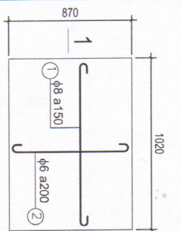
TẦM ĐÀN D1 (SL = 02C.K) TỈ LỆ : 1/25
