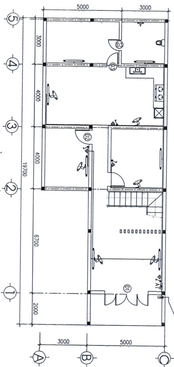
MẶT BẰNG CẤP ĐIỆN TẦNG 1
