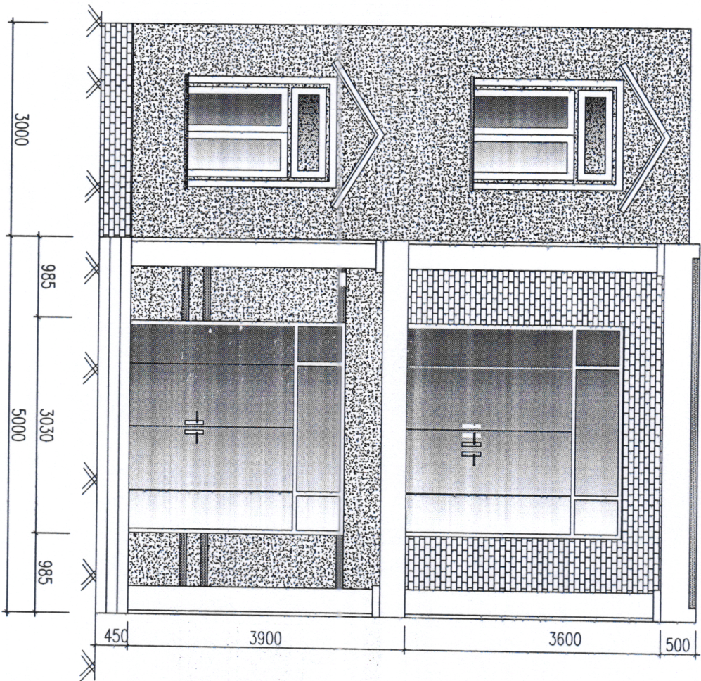
MẶT ĐÚNG CHÍNH (TL: 1/100)
