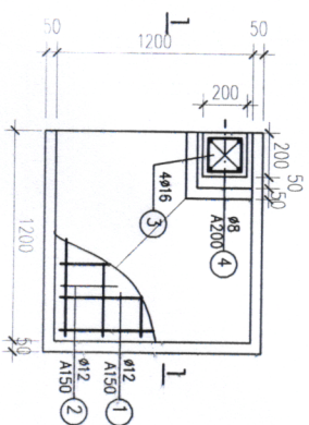
MŨNG TRỪ MC2 (SL: 02CK)
