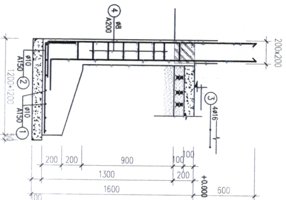
CẮT 1-1
