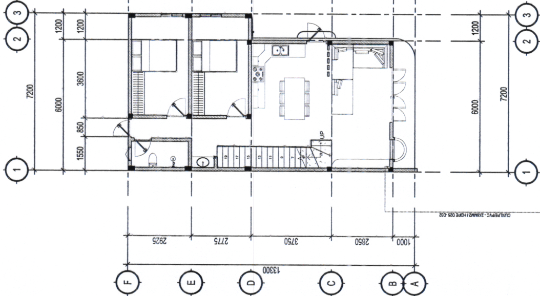
MẶT BẰNG CẤP ĐIỆN TẦNG 1 TỶ LỆ 1/100
