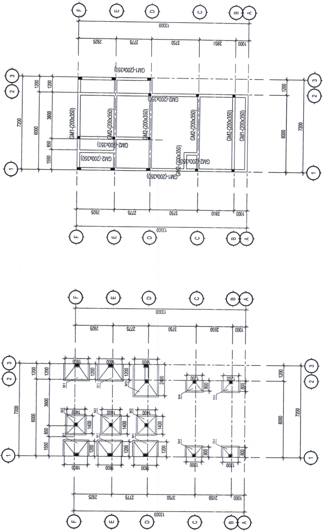
MẶT BẰNG GIẢNG MÓNG TỶ LỆ 1/100
