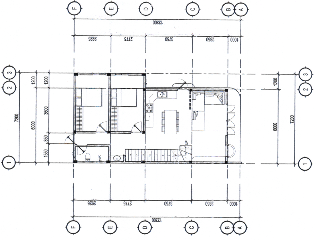
MẶT BẰNG TẦNG 1 TỶ LỆ 1/100
