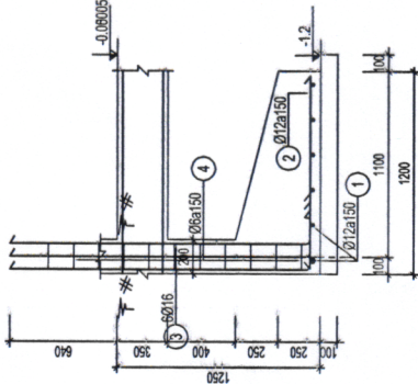
MẶT CẮT B-B
