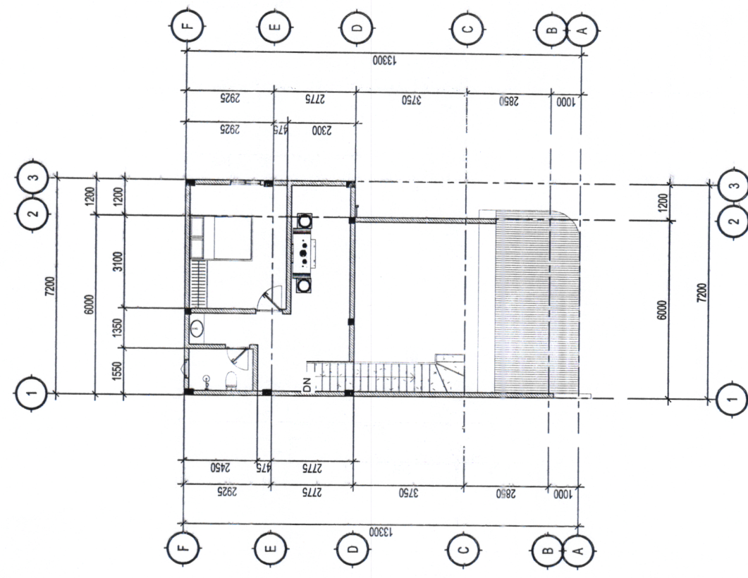
MẶT BẰNG TẦNG 2 TỶ LỆ 1/100
