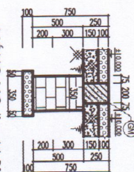
MÔNG MG (L = 14.3M) TỈ LỆ: 1/25
