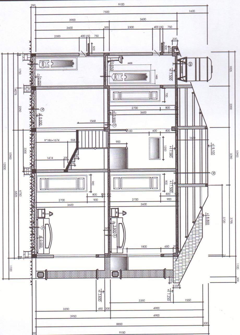
MẶT CẮT C-C
