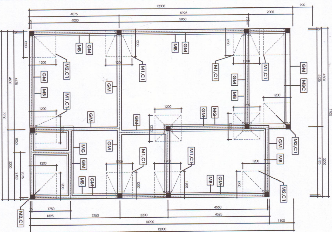
MẶT BẰNG MÔNG TỈ LỆ: 1/50
