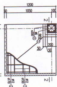
MÔNG M2 (05 CK) TỈ LỆ: 1/25
