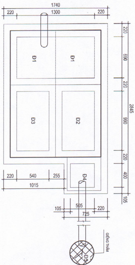
MẶT BẰNG BỐ TRÍ ĐÀN
