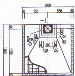
MÔNG M1 (05 CK) TỈ LỆ: 1/25
