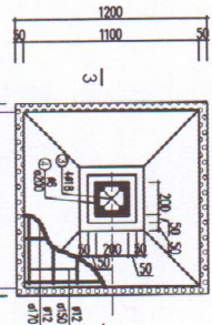
MÔNG M3 (02 CK) TỈ LỆ: 1/25
