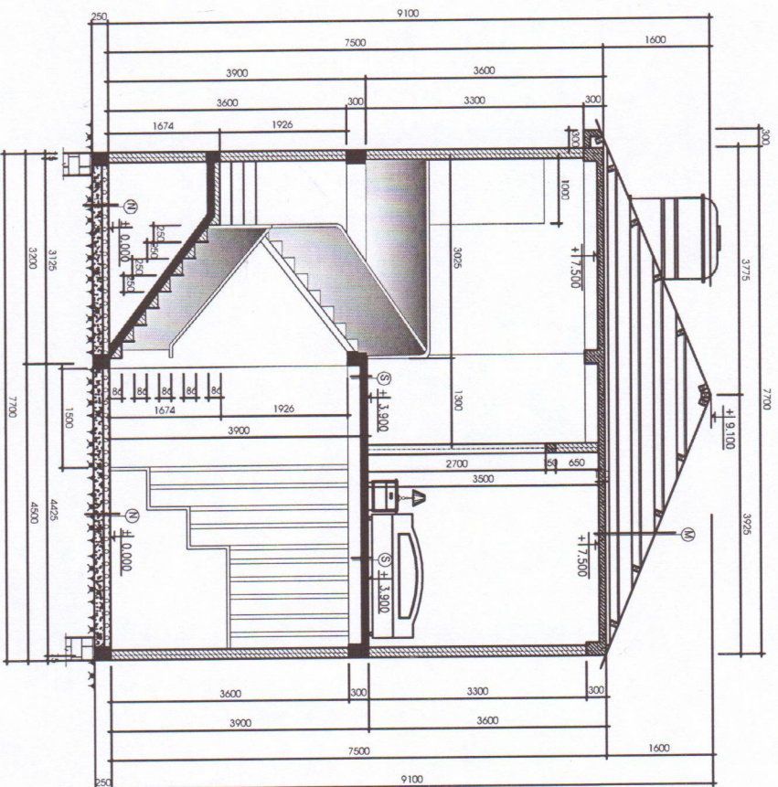
MẶT CẮT D-D
