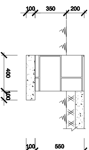
MẶT CẮT 1-1
