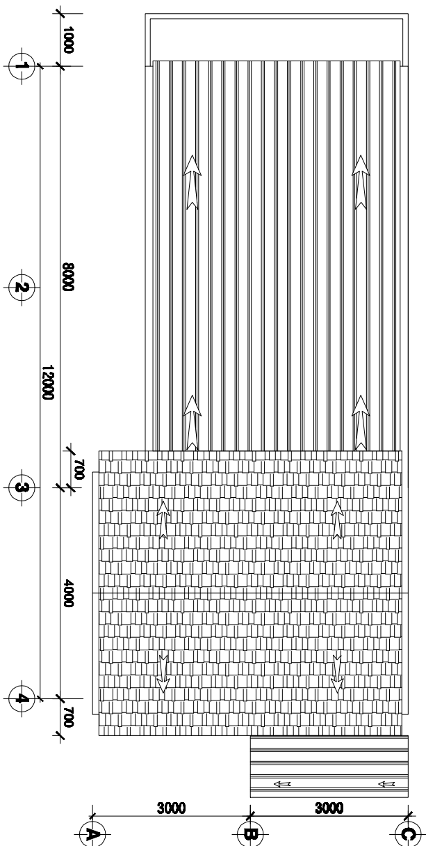
MẶT BẰNG Mái ( TL 1:100)
