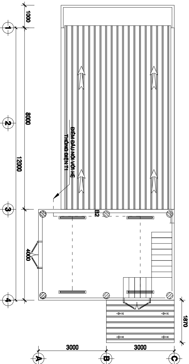
MẶT BẰNG CẤP ĐIỆN T2 (TL 1:100)
