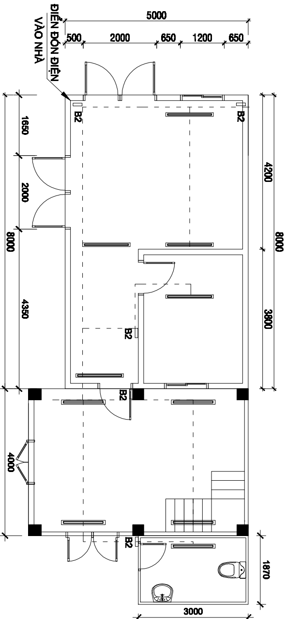
MẶT BẰNG CẤP ĐIỆN T1 (TL 1:100)
