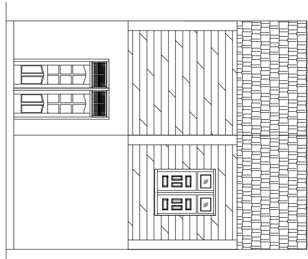
MẶT ĐỨNG TRỤC A-C ( TL 1:100)
