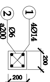
MẶT CẮT 1-1
