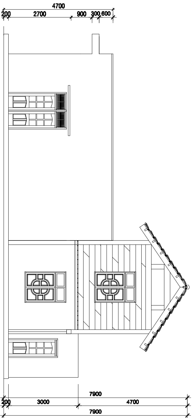
MẶT BÊN TRỤC 1-4 ( TL 1:100)
